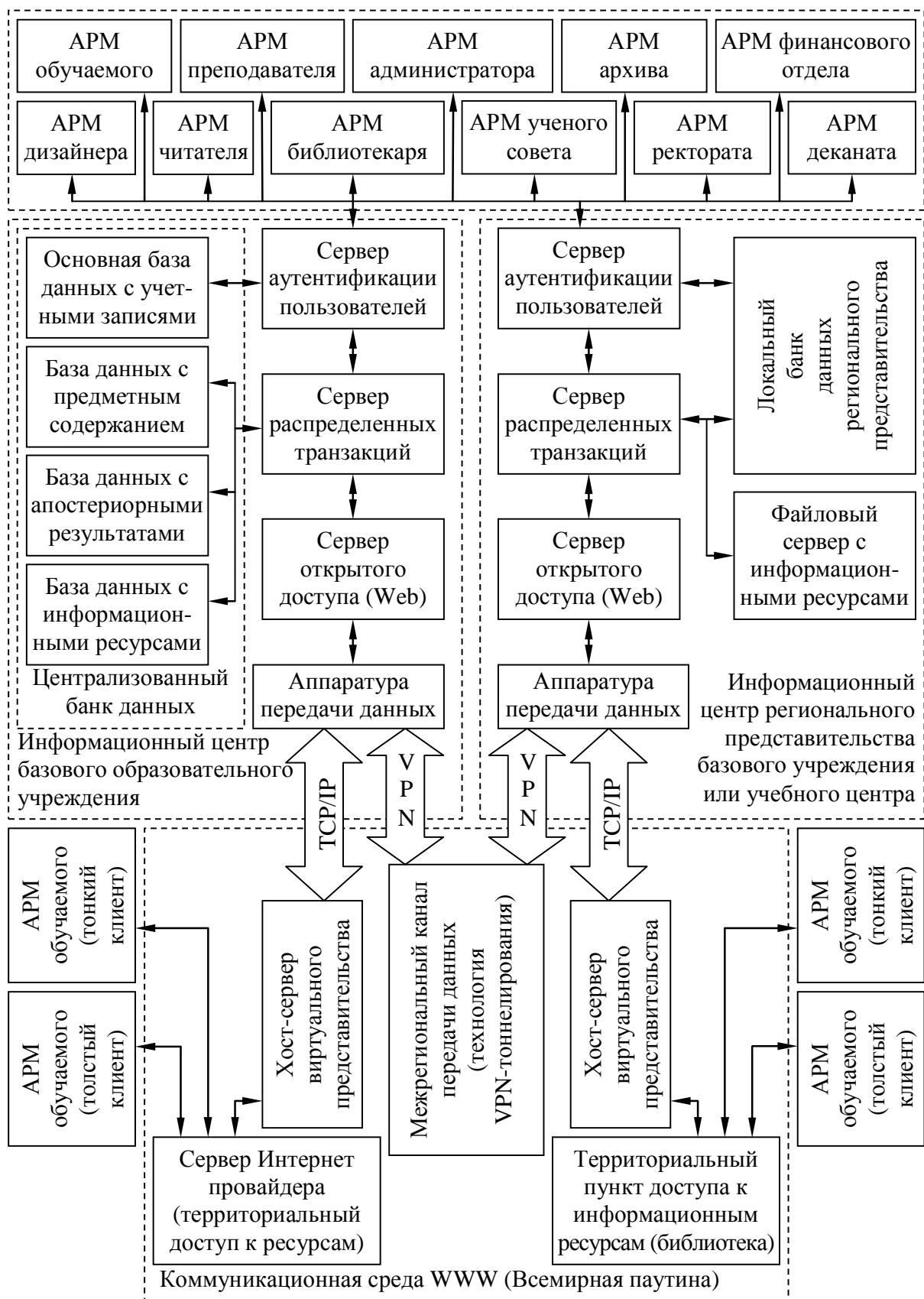
Рис. 2.12. Типовая схема взаимодействия информационного центра образовательного учреждения и автоматизированных рабочих мест Информационная среда учреждений включает АРМ и поддерживается информационными центрами, предоставляющими доступ к ресурсам глобальных и ЛВС.
