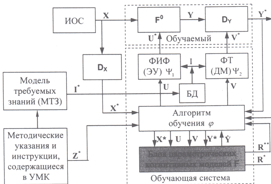
Рис. 1. Структурная схема системы обучения на основе когнитивных моделей
