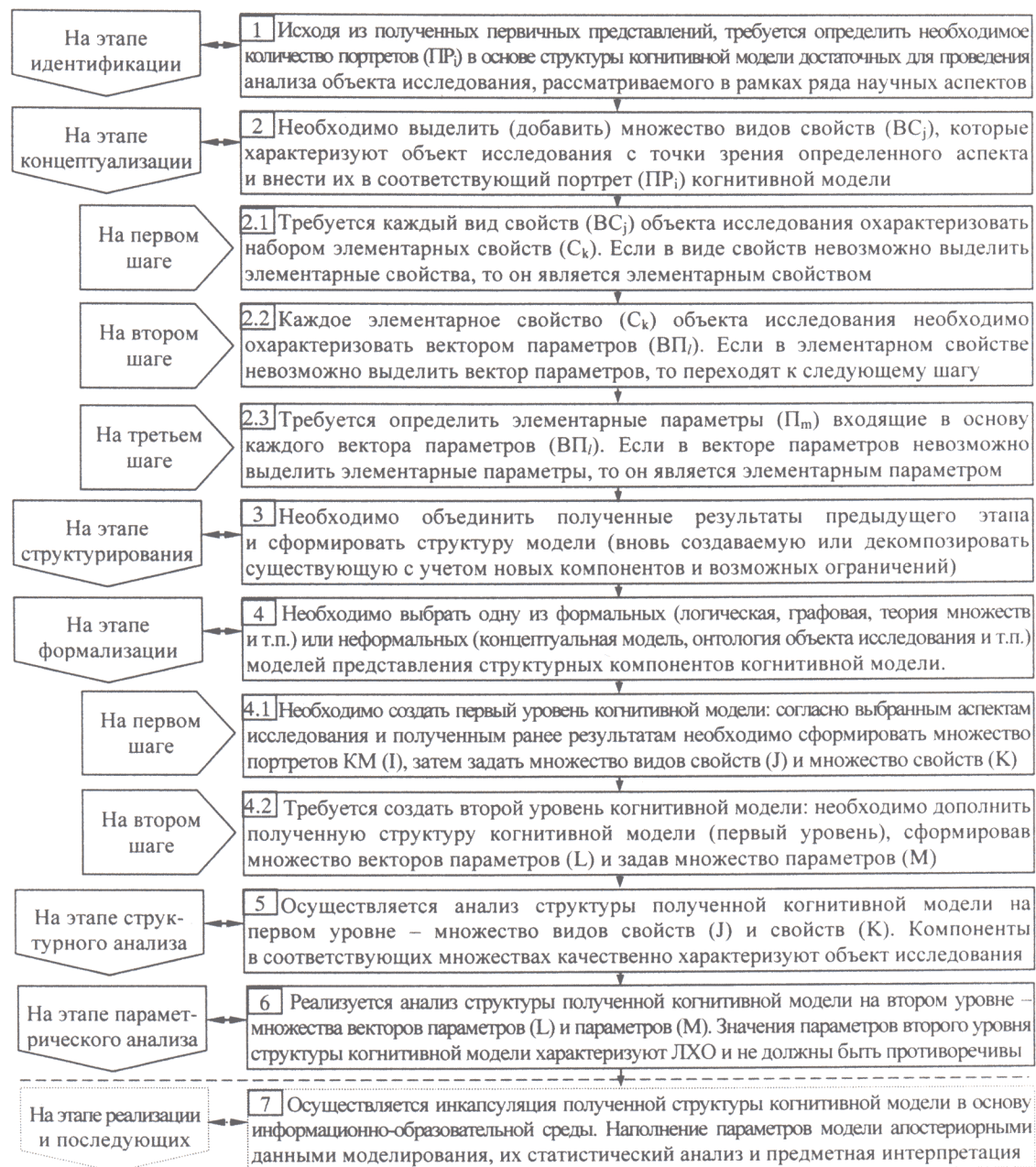
Рис. 5. Алгоритм формирования структуры когнитивной модели
