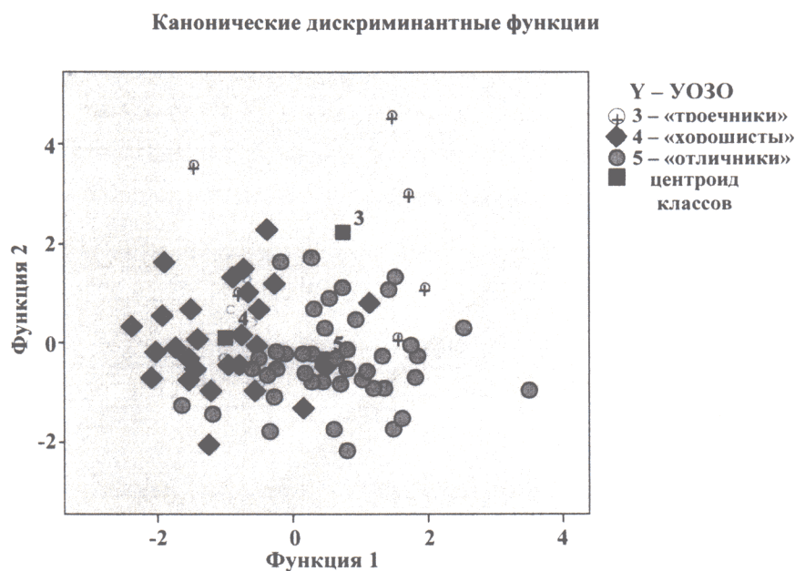
Рис. 13. Центроиды классов обучаемых в пространстве канонических функций
