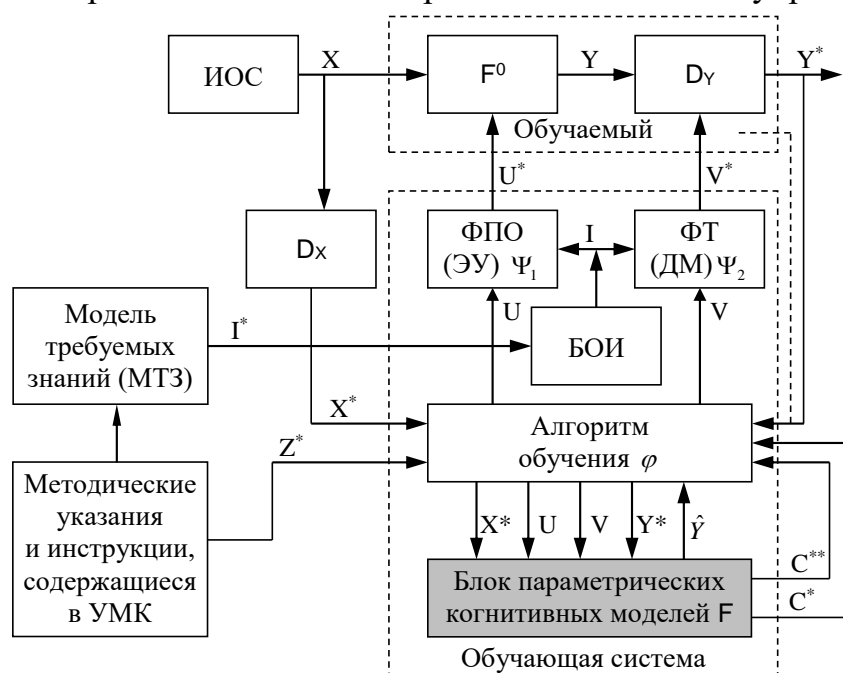
Рисунок 4. Структурная схема системы АДО с элементами адаптации на основе блока параметрических когнитивных моделей
