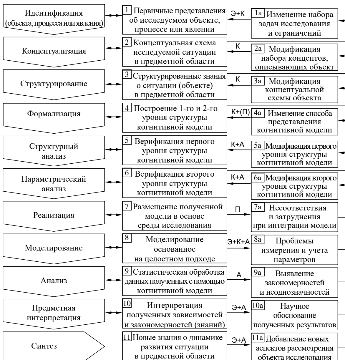
Рисунок 5. Итеративный цикл технологии когнитивного моделирования
